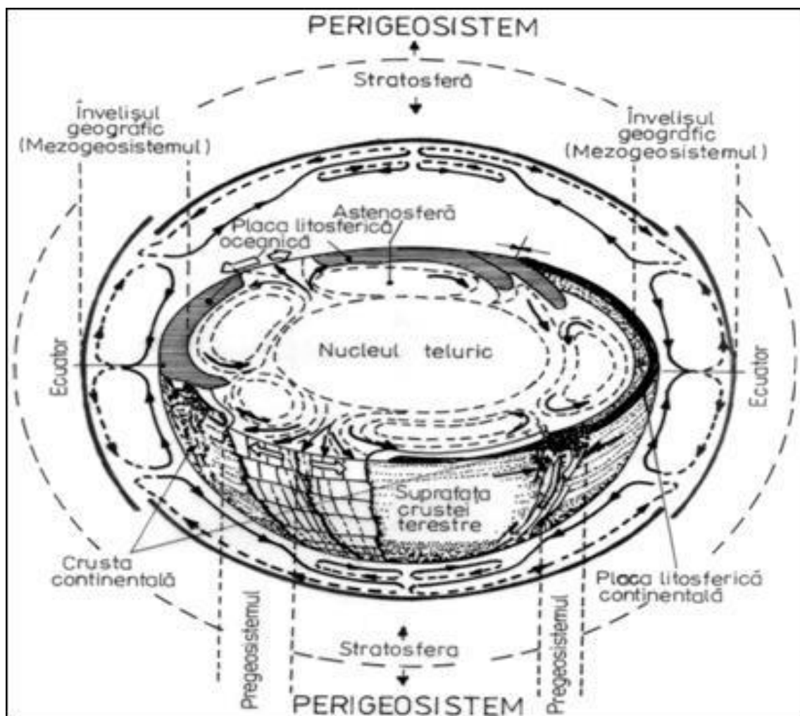
Fig. 1. Poziționarea telurică a învelișului geografic (după Al. Rosu, 1987).
